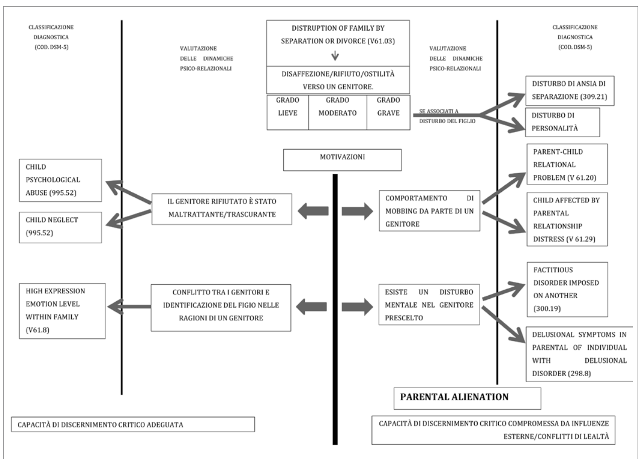
Fig. 1. Algoritmo valutativo.
